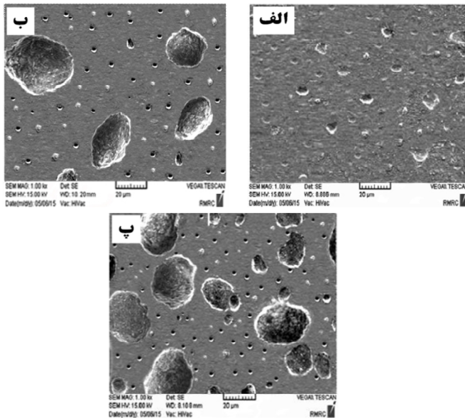
شکل ۹- تصاویر SEM از سطح خوردگی: الف) فلز پایه، ب) فلز جوش ایجاد شده با حرارت ورودی 6/75 \text{ J/mm} ، پ) فلز جوش ایجاد شده با حرارت ورودی 11/25 \text{ kJ/mm}
