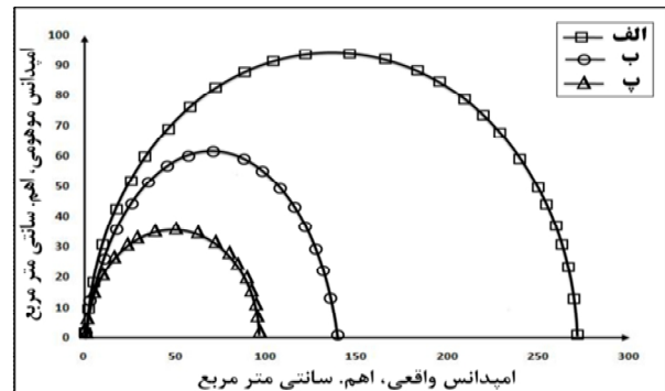
شکل ۷- نمودار نایکوئیست مربوط به آزمایش طیف سنجی امپدانس الکتروشیمیایی در حداقل سه بار تکرارپذیری: الف) فلز پایه، ب) فلز جوش ایجاد شده با حرارت ورودی 6/75 \text{ kJ/mm} ، پ) فلز جوش ایجاد شده با حرارت ورودی 11/25 \text{ kJ/mm}
