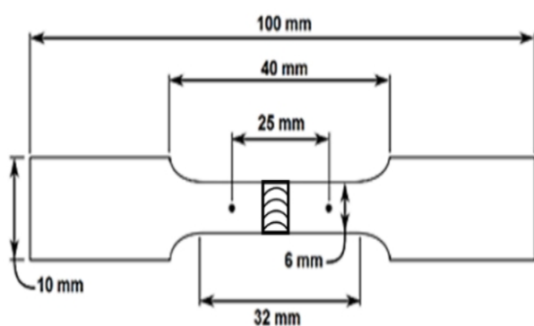
شکل ۱- ابعاد نمونه کشش بر اساس استاندارد ASTM.E8/E8M
