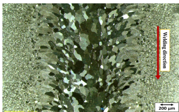
شکل ۶- تصویر دانه بندی روی جوش پرتو الکترونی آلیاژ Nb-1Zr
