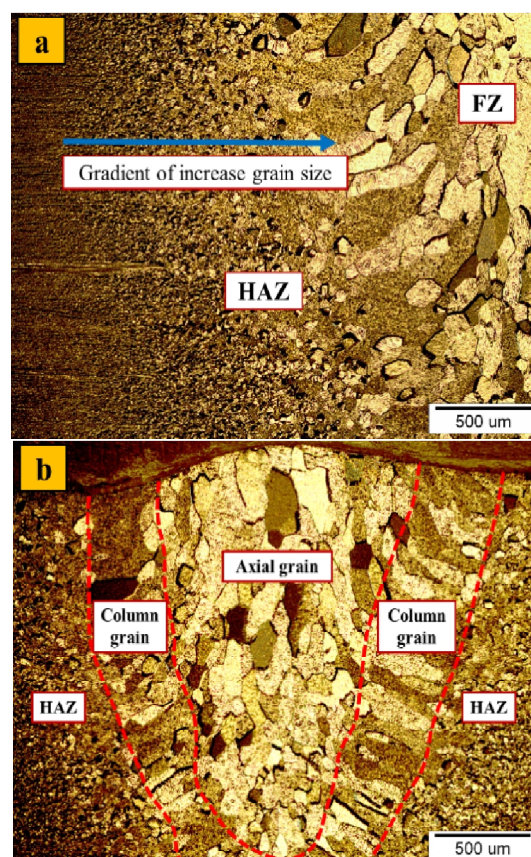
شکل ۵- ساختار میکروسکوپی مناطق جوشکاری پرتو الکترونی نمونه N2 توسط میکروسکوپ نوری.
