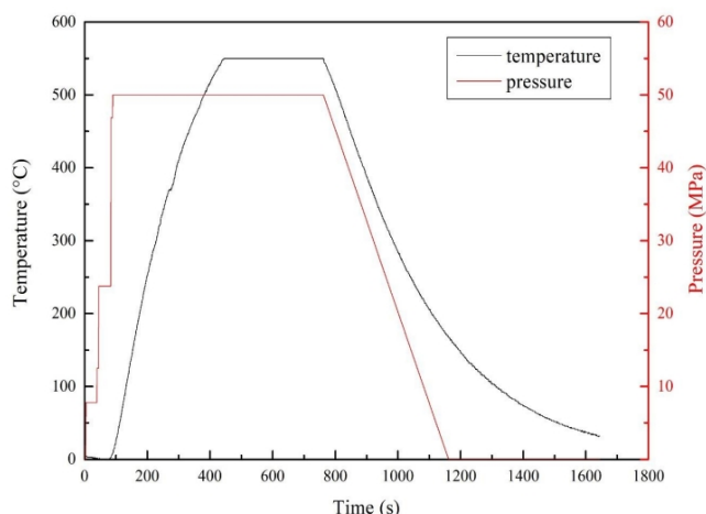
شکل 1- دما و فشار اعمال شده طی فرایند قوس الکتریکی پلاسما.
