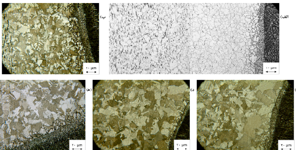
شکل ۱۱- ریزساختار ناحیه HAZ: (الف) H1، (ب) H2، (ج) MIG1، (د) MIG2 و (ه) TIG.
