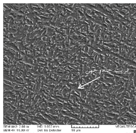
شکل 9 - تصاویر میکروسکوپی الکترونی روبشی با بزرگنمایی برابر از ریزساختار منطقه جوش. اعداد زیر هر تصویر مربوط به شرایط اعمال شده طبق جدول 6 می باشد. (اج شده با محلول نایتال 2%)
