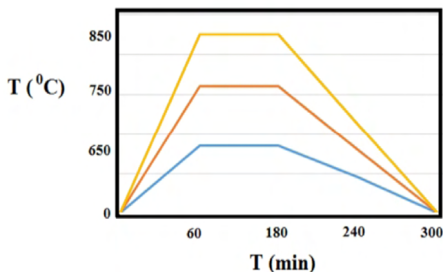
شکل 1- شماتیک نحوه اجرای عملیات حرارتی
