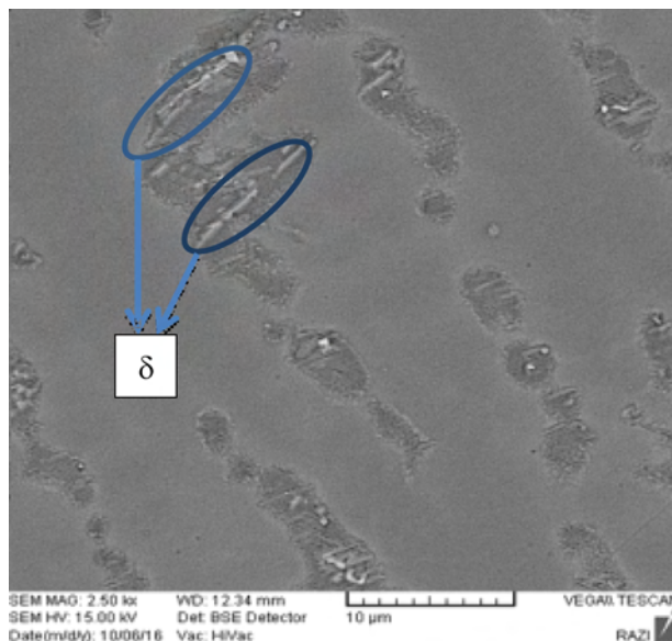
شکل 5- فاز \delta تشکیل شده در 750 درجه سانتیگراد
