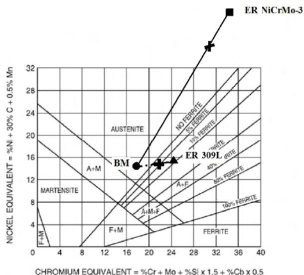
شکل 1- پیش‌بینی ساختار فلزپایه و فلزپرکننده \times ، به ترتیب معرفی
