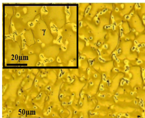
شکل 2- ریزساختار نوری فلزپایه (الف) و فلزجوش راسب شده از
