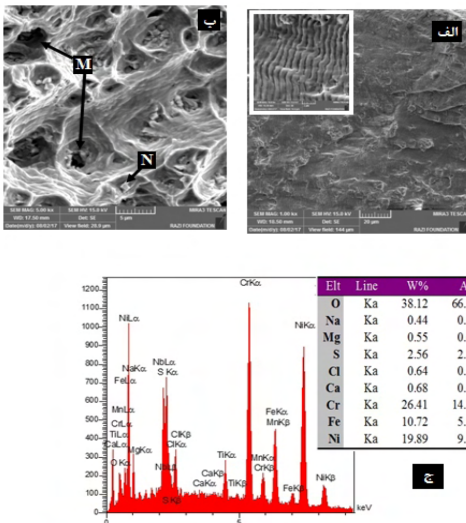
شکل 10- مطالعه سطح شکست خوردگی -خستگی نمونه جوشکاری شده با فلز پرکننده ERNiCrMo-3. (الف) سطح شکست، (ب) تشکیل حفرات و محصولات غنی از محیط خورنده، (ج) آنالیز EDS از ذرات M و N به ترتیب معرف حفرات و محصولات خوردگی در سطح شکست می باشد.
