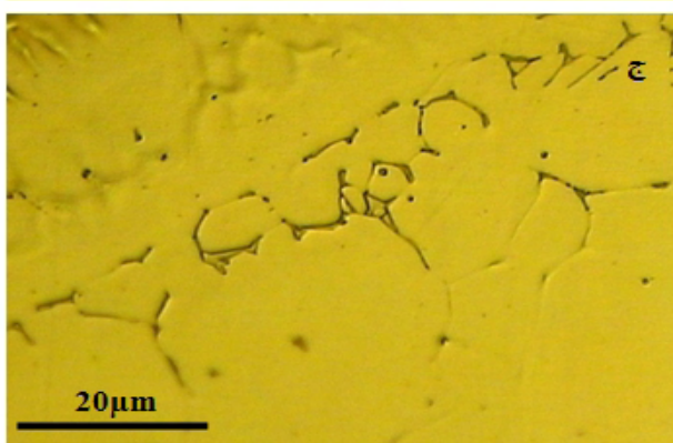
شکل 4- الف) ساختار نوری نرمال فصل مشترک WM/HAZ.
