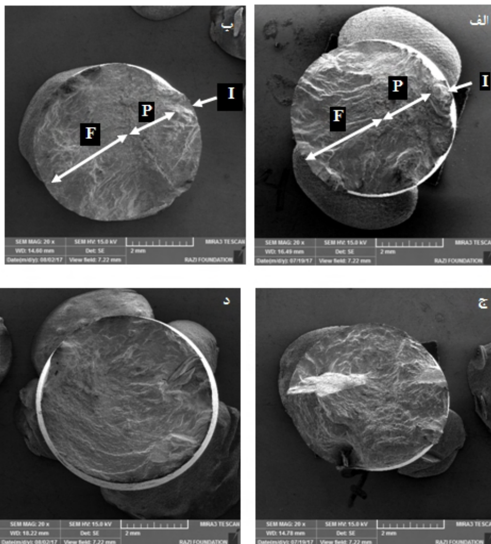
شکل 7- مطالعه میکروسکوپی سطوح شکست نمونه‌های خستگی (الف و ب) و خوردگی-خستگی (ج و د). نمونه‌های جوشکاری شده با فلزپرکننده ER309L (الف و ج) و جوشکاری شده با فلزپرکننده ERNiCrMo-3 (ب و د). علائم F و P به ترتیب معرف محل ایجاد ترک، منطقه اشاعه ترک و موضع شکست نهایی می‌باشد.
