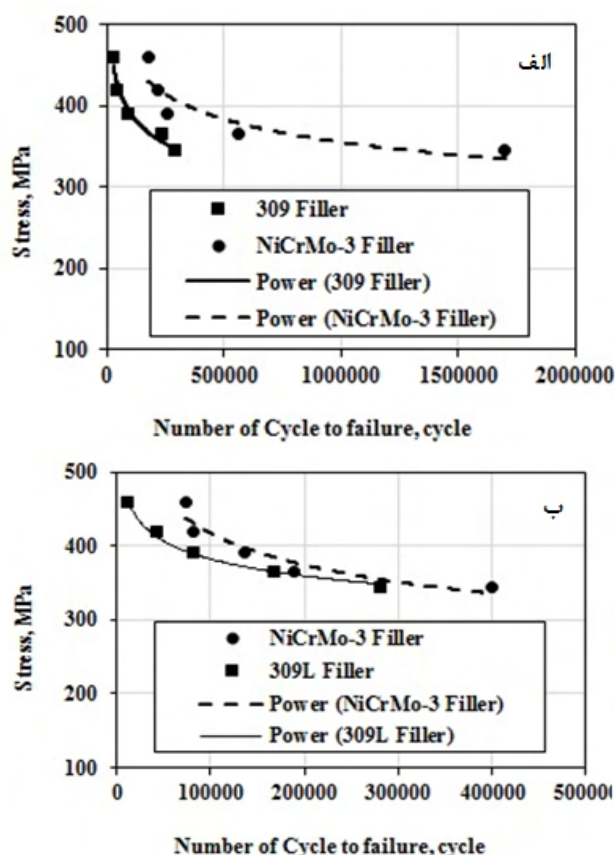
شکل 6- تاثیر فلزپرکننده بر رفتار فلزجوش در آزمونهای (الف) خستگی، (ب) خوردگی-خستگی.
