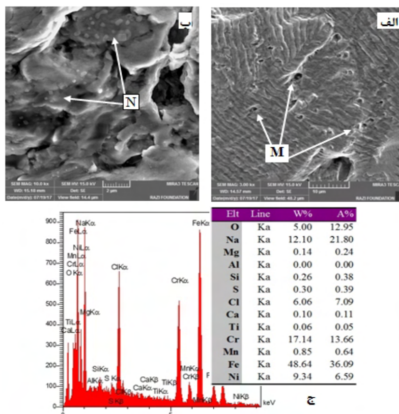
شکل 9- مطالعه سطح شکست خوردگی-خستگی نمونه جوشکاری شده با فلزپرکننده ER309L. (الف) تشکیل حفرات، (ب) تشکیل محصولات غنی از محیط خورنده، (ج) آنالیز EDS از ذرات M و N به ترتیب معرف حفرات و محصولات خوردگی در سطح شکست می‌باشد.
