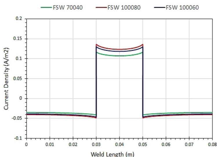
شکل 6- نتایج حاصل از شبیه سازی توزیع جریان خوردگی گالوانیکی در عرض مقطع جوش لوله برای نمونه های جوشکاری شده به روش الکترو تنگستنی.
