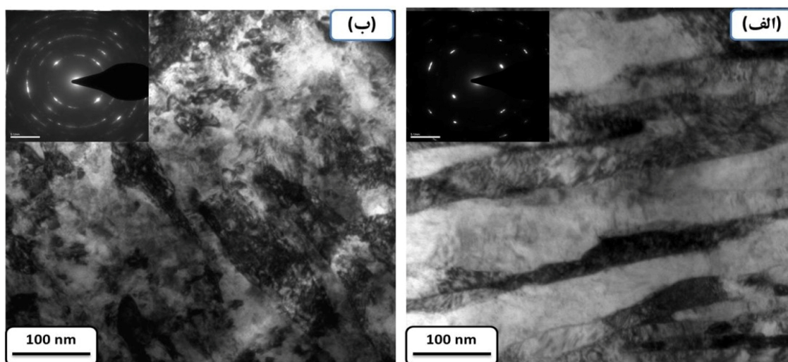
شکل ۴-تصاویر میکروسکوپی الکترونی عبوری از ریزساختار فولاد زنگ زن ۳۰۴ L پس از ۸۰٪ نورد سرد
