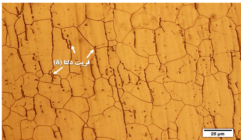
شکل ۳-ریزساختار فولاد زنگ زن ۳۰۴ L درشت دانه
