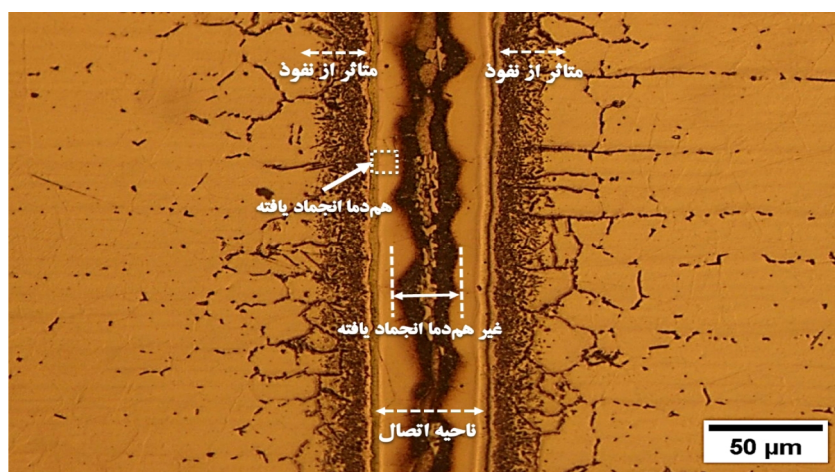
شکل ۵- ناحیه اتصال فولاد زنگ نزن L ۳۰۴ درشت دانه در زمان ۵ دقیقه و دمای ۱۰۵۰°C
