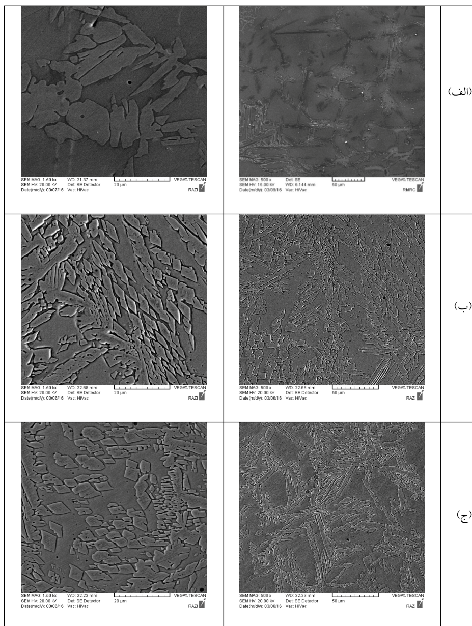
شکل 4- تصاویر میکروسکپی الکترونی روبشی از منطقه‌ی جوش نمونه‌های حاصل از جوشکاری در حرارت‌های ورودی (الف) 0/6، (ب) 1/0 و (ج) 1/4 کیلوژول بر میلی‌متر.
