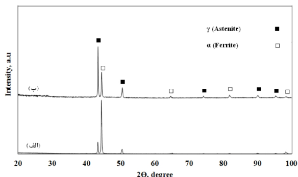
شکل 6- الگوهای پراش پرتو ایکس مربوط به منطقه‌ی جوش نمونه‌های حاصل از جوشکاری در حرارت‌های ورودی (الف) 0/6 ، (ب) 1/4 کیلوژول بر میلی‌متر.
