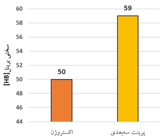
شکل 8- مقایسه میانگین سختی برینل برای نمونه‌های اکستروژن و پرینت سه‌بعدی.
