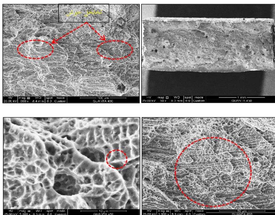
شکل 11- تصاویر میکروسکوپ الکترونی روبشی از سطح شکست آزمون کشش در دمای محیط فلز جوش نمونه شماره 9.
