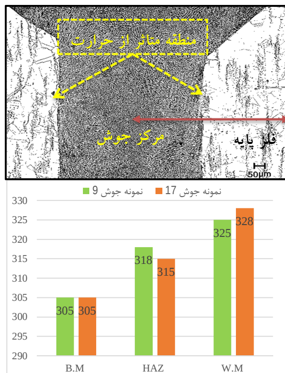
شکل 8- الف - مقطع عرضی جوش نمونه شماره 17، ب - نمودار ریزسختی منطقه جوش، منطقه تحت تاثیر حرارت و فلز پایه نمونه‌های 9 و 17.
