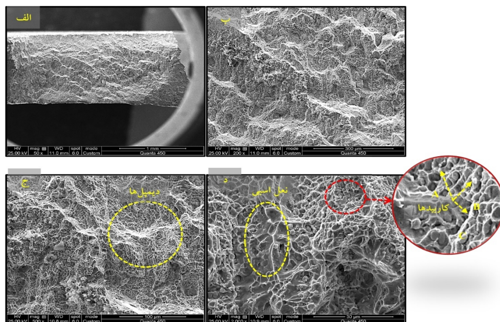
شکل 10- تصاویر میکروسکوپ الکترونی روبشی از سطح شکست نمونه آزمون کشش در دمای محیط فلز پایه و تحلیل طیف سنجی انرژی پراش پرتو ایکس از کاریدهای موجود در سطح.
