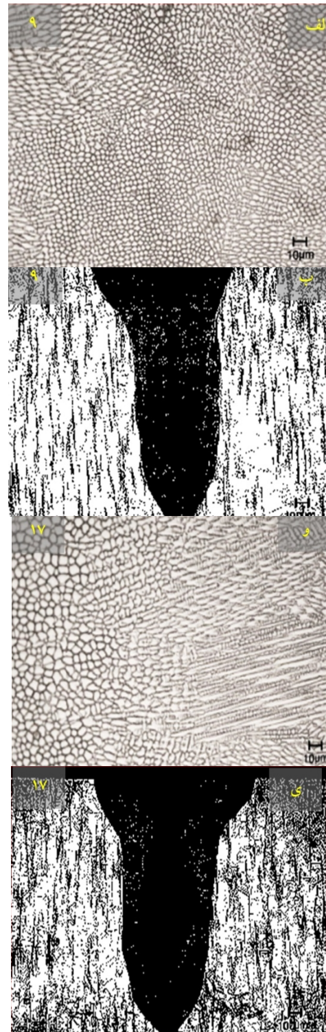
شکل 5- تصاویر میکروسکوپ نوری سطح و مقطع عرضی و ریزساختار منطقه جوش الف، ب- نمونه 9 و و، ی- نمونه 17.
