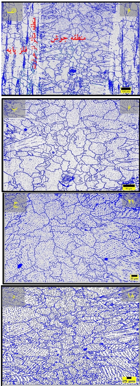
شکل 3- تصاویر ریزساختاری نمونه‌های جوش داده شده الف- فلز پایه و فلز جوش شماره 6، ب- مرکز جوش شماره 6، ج- مرکز جوش شماره 21، د- مرکز جوش شماره 18.
