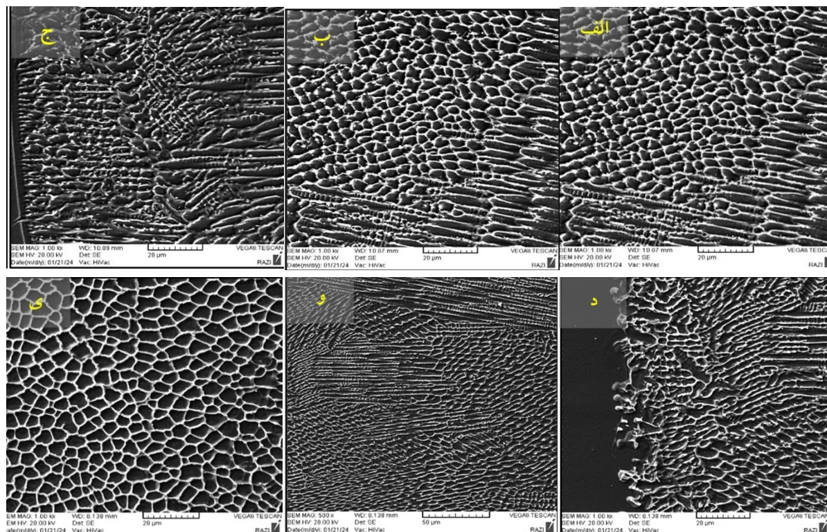
شکل 6- تصاویر میکروسکوپ الکترونی روبشی (SEM) ریزساختار الف، کناره جوش ب، تا وسط آن جوش نمونه
