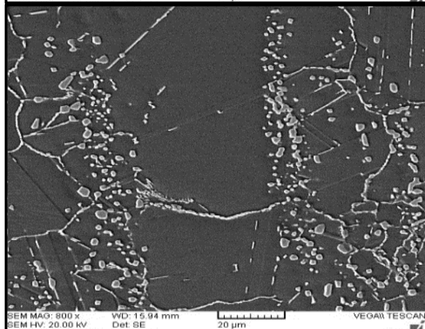
شکل 1- تصاویر میکروسکوپ الکترونی روبشی برای ابرآلیاژ هاینس 25
