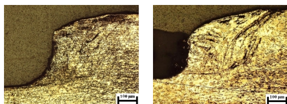
شکل 7- تصویر میکروسکوپی کنار جوش نمونه با مدت زمان تماس 40 ثانیه و سرعت دورانی 1320 (الف)، 1800 (ب) و 2500 (پ)
