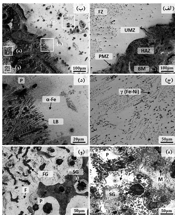
شکل 6- تصاویر میکروسکوپی نوری از نواحی مختلف چدن خاکستری جوشکاری شده به روش SMAW با الکترود ENi-CI: الف و ب- فصل مشترک FZ و FZ، ج- FZ، د- UMZ و HAZ و، و- BM.
