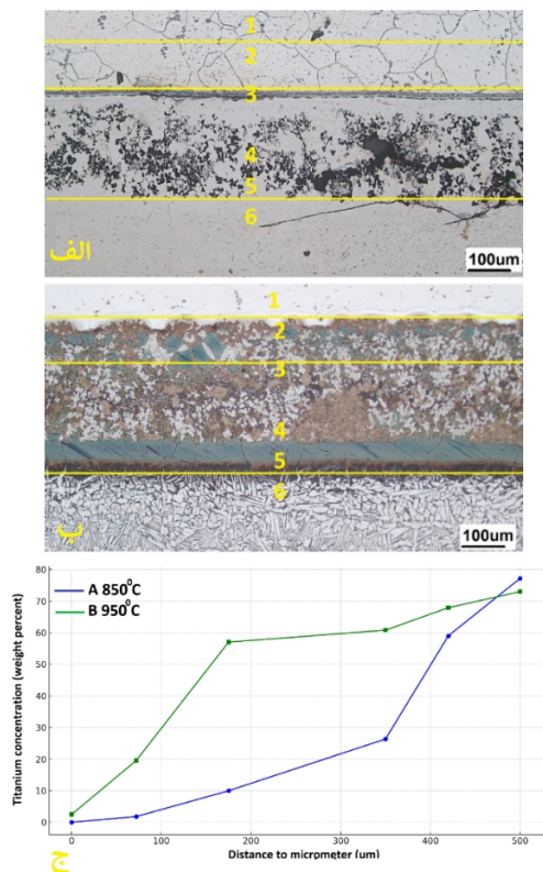
شکل 12- اثر توزیع عنصر تیتانیوم بر روی ریزساختار اتصال فرایند TLP در دمای: الف - 850 درجه سانتی گراد، ب - 950 درجه سانتی گراد و ج - نمودار توزیع عنصر تیتانیوم در دو ریزساختار.
