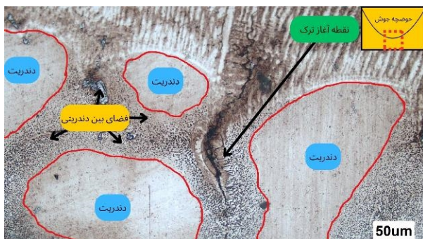
شکل 10- محل آغاز ترک در نمونه 1A-GTAW گرم بر میلی لیتر از فضای بین دندریت ها بوده است.
