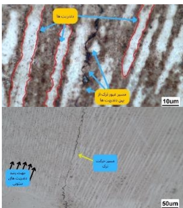
شکل 11- مسیر حرکت ترک نمونه بهینه 1A-GTAW گرم بر میلی لیتر زیگزاگی و از میان دندریت بوده ها که از مشخصه های ترک ذوبی است.
