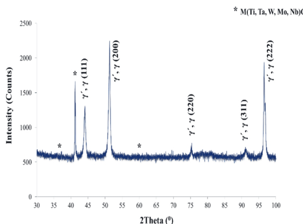
شکل 8- نمودار XRD از تک پاس‌های IN738LC.
