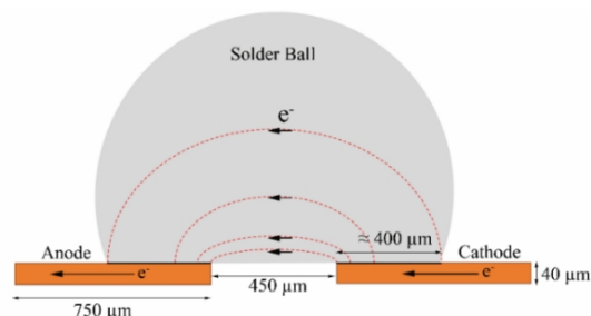
شکل 3- تصویر شماتیک آزمون مهاجرت الکترون.
