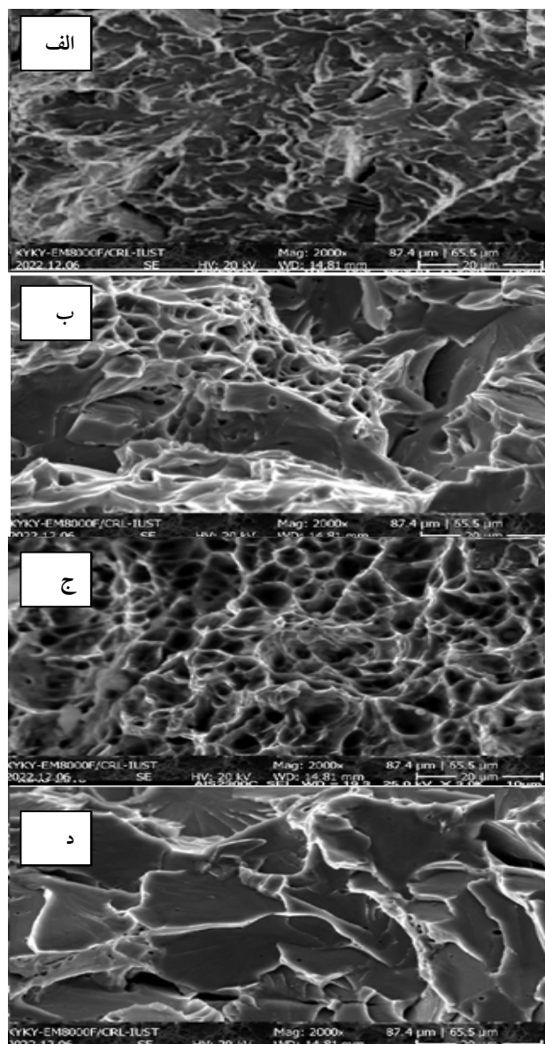
شکل ۱۱- تصاویر میکروسکوپ الکترونی روبشی از سطح شکست نمونه‌های
