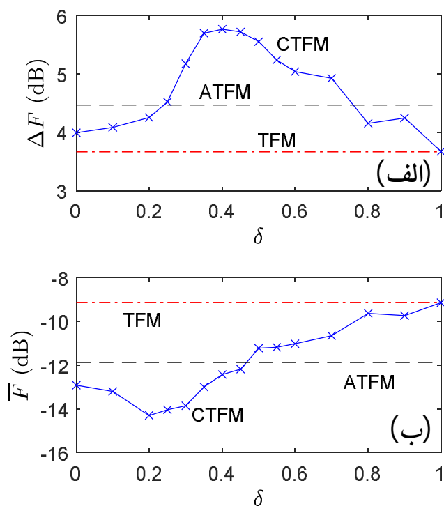
شکل 8- نمودار تابع \Delta F (شکل الف) و تابع \bar{F} (شکل ب) بر حسب \delta برای روش CTFM به همراه مقدار آن برای TFM و ATF.
