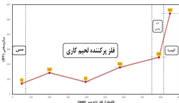
شکل 18- نمودار ریزسختی ویکرز اتصال آلومینا به مس با فلز پرکننده \text{Ag-Cu-Ti-Sn-}\%3.5\text{Zr} برحسب فاصله.
