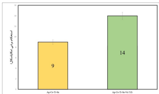
شکل 16- نتایج آزمون استحکام برشی اتصالات لحیم کاری.
