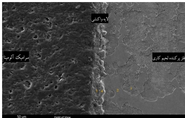
شکل 8- تصویر میکروسکوپی الکترونی روبشی از اتصال لحیم کاری \text{Al}_2\text{O}_3/\text{Cu} با فلز پرکننده Ag-Cu-Ti-Sn.
