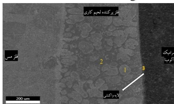
شکل 12- تصویر میکروسکوپی الکترونی روبشی از اتصال \text{Al}_2\text{O}_3/\text{Cu} با فلزپرکننده \text{Ag-Cu-Ti-Sn-3.5Zr} .
