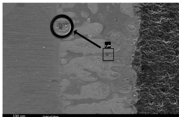
شکل 11- تصویر میکروسکوپی الکترونی روبشی از اتصال \text{Al}_2\text{O}_3/\text{Cu} با فلز پرکننده Ag-Cu-Ti-Sn.
