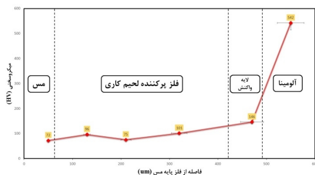
شکل 17- نمودار ریزسختی ویکرز اتصال آلومینا به مس با فلز پرکننده \text{Ag-Cu-Ti-Sn} برحسب فاصله.
