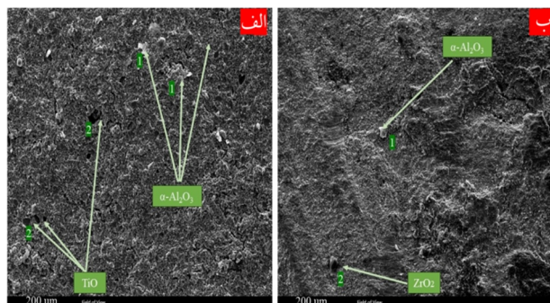
شکل 19- تصاویر SEM از سطوح شکست اتصالات لحیم کاری با فلزات پرکننده \text{Ag-Cu-Ti-Sn} (الف) و \text{Ag-Cu-Ti-Sn-}\%3.5\text{Zr} (ب).
