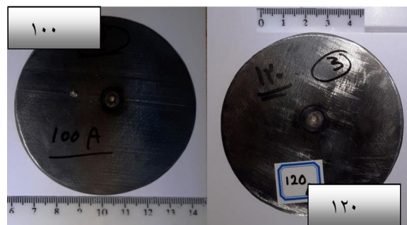
شکل 5- نمونه های جوشکاری شده با شدت جریان های 100 و 120 آمپر.
