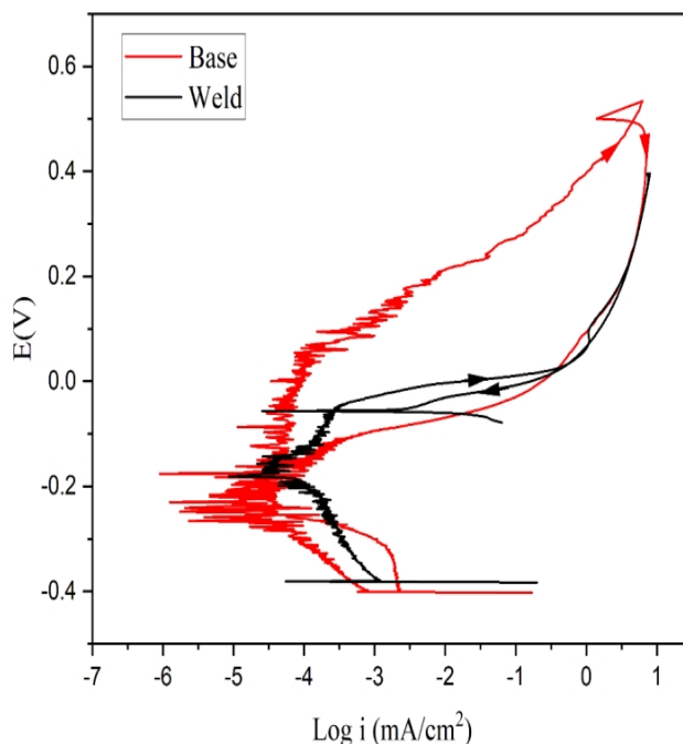
شکل 2- نمودار پلاریزاسیون مربوط به فلزجوش (رنگ مشکی) و فلزپایه (رنگ قرمز) در محلول 3/5% NaCl.
