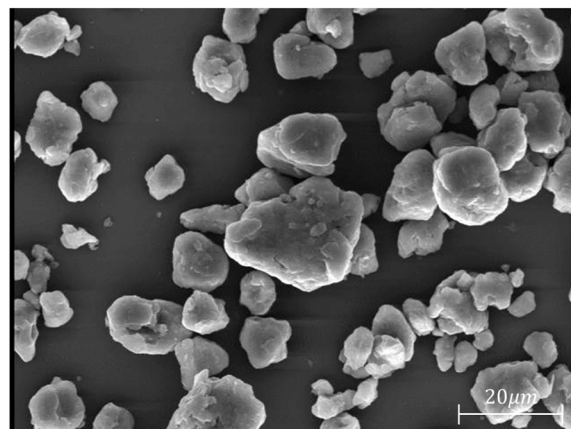
شکل 7- میکروگراف ذرات آلومیناید مولیدن. اندازه‌ی میانگین ذرات در حد 20 \mu m است (اندازه گیری با ImageJ).
