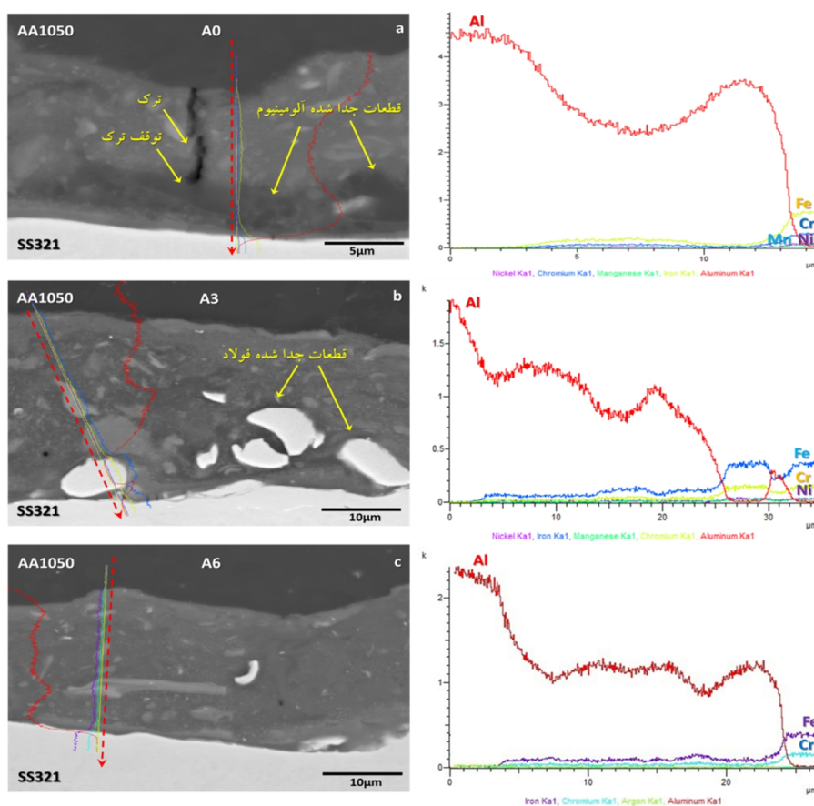
شکل 2- تصویر میکروسکوپ الکترونی و توزیع خطی عناصر در لایه واکنشی در فصل مشترک اتصال 3 لایه Al1050-SS312 نمونه‌های سری A (فاصله کاری A0، A3 و A6 به ترتیب 14/5، 12/9 و 13/0 میلی متر، شناساگر الکترون برگشتی)
