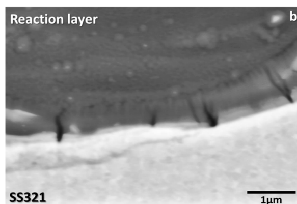
شکل 4- تصویر میکروسکوپ الکترونی ریزترک‌ها در مرز فولاد با لایه واکنشی (فاصله کاری 7/9 میلی‌متر، شناساگر الکترون برگشتی)
