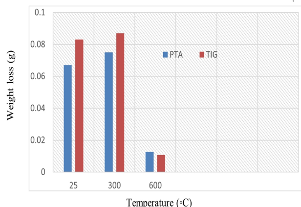
شکل 13- مقایسه کاهش جرم در روکش قوس تنگستن و قوس پلاسما در دماهای مختلف
