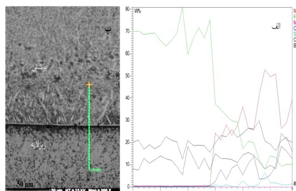
شکل 7- آنالیز خطی از مقطع روکش آلیاژ کلمونوی جوشکاری شده به روش قوس تنگستنی، الف- نفوذ عناصر در فصل مشترک و ب- فصل مشترک روکش
