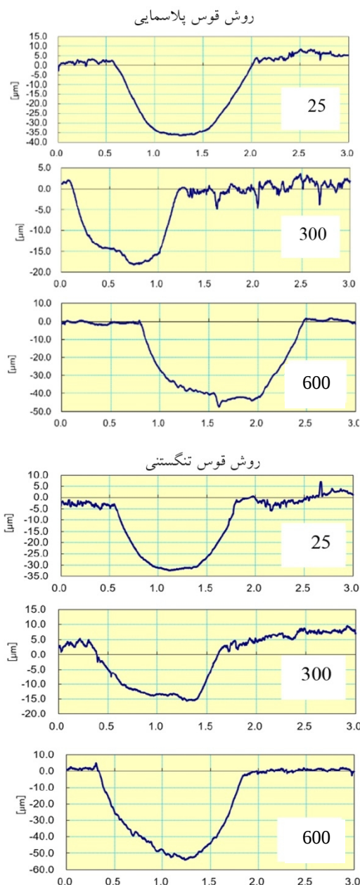
شکل 12- بررسی عمق سایش در دو روش روکش کاری قوس تنگستن و قوس پلاسما در دماهای مختلف: دمای اتاق، 300 و 600 درجه. در دمای 600 درجه عمق ساییده شده به مراتب بیشتر است.
