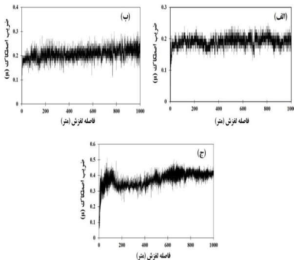
شکل 20- نمودار تغییرات ضریب اصطکاک بر حسب مسافت لغزش برای روکش (Fe, Cr)_3Al در دماهای، الف - 25 °C، ب - 200 °C و ج - 500 °C
