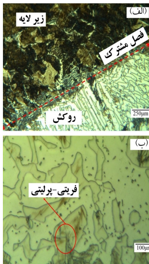
شکل 4- ریزساختار سطح مقطع پوشش Fe_3Al (الف) ریزساختار فصل مشترک پوشش/زیرلایه و (ب) ریزساختار پوشش Fe_3Al .
