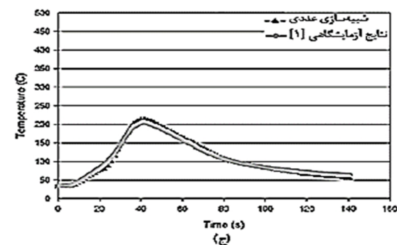
شکل 4- نتایج شبیه‌سازی عددی و نتایج آزمایشگاهی در قطعه کار و مقایسه آن با دمای پیش‌بینی شده در سرعت دورانی 350 دور بر دقیقه و سرعت پیشروی ابزار 3 میلی‌متر بر ثانیه و در سه فاصله مختلف، الف- 7 میلی‌متر، ب- 15 میلی‌متر، ج- 25 میلی‌متر از خط جوش.
