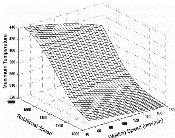
شکل 7- تاثیر همزمان سرعت چرخش و سرعت خطی بر دمای بیشینه در نقطه‌ای به فاصله 7 میلی‌متر از خط جوش
