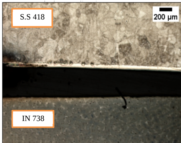
شکل 15- تصویر میکروسکوپ نوری نمونه S8 در بزرگمایی 5X.
