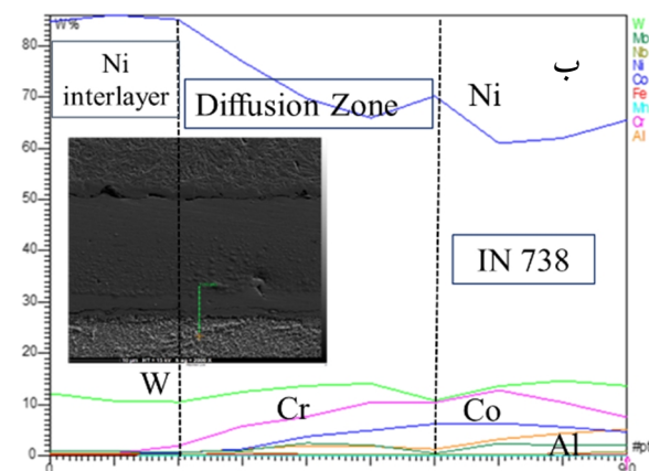
شکل 14- آنالیز اسکن خطی نمونه S7 در الف - سمت فولاد مارتنزیتی 418 ب - سوپرآلیاژ اینکونل 738.
