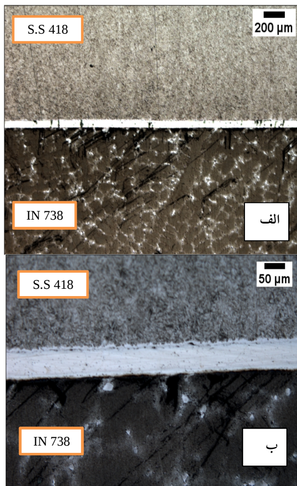
شکل 5- تصویر میکروسکوپ نوری نمونه S5 در بزرگنمایی
