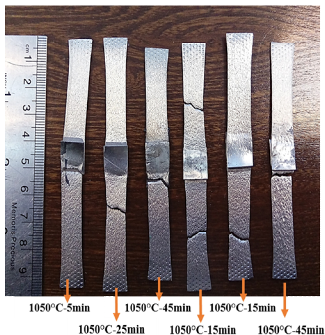
شکل 9. نمونه های اتصال داده شده اینکونل 600 بعد از آزمون استحکام
