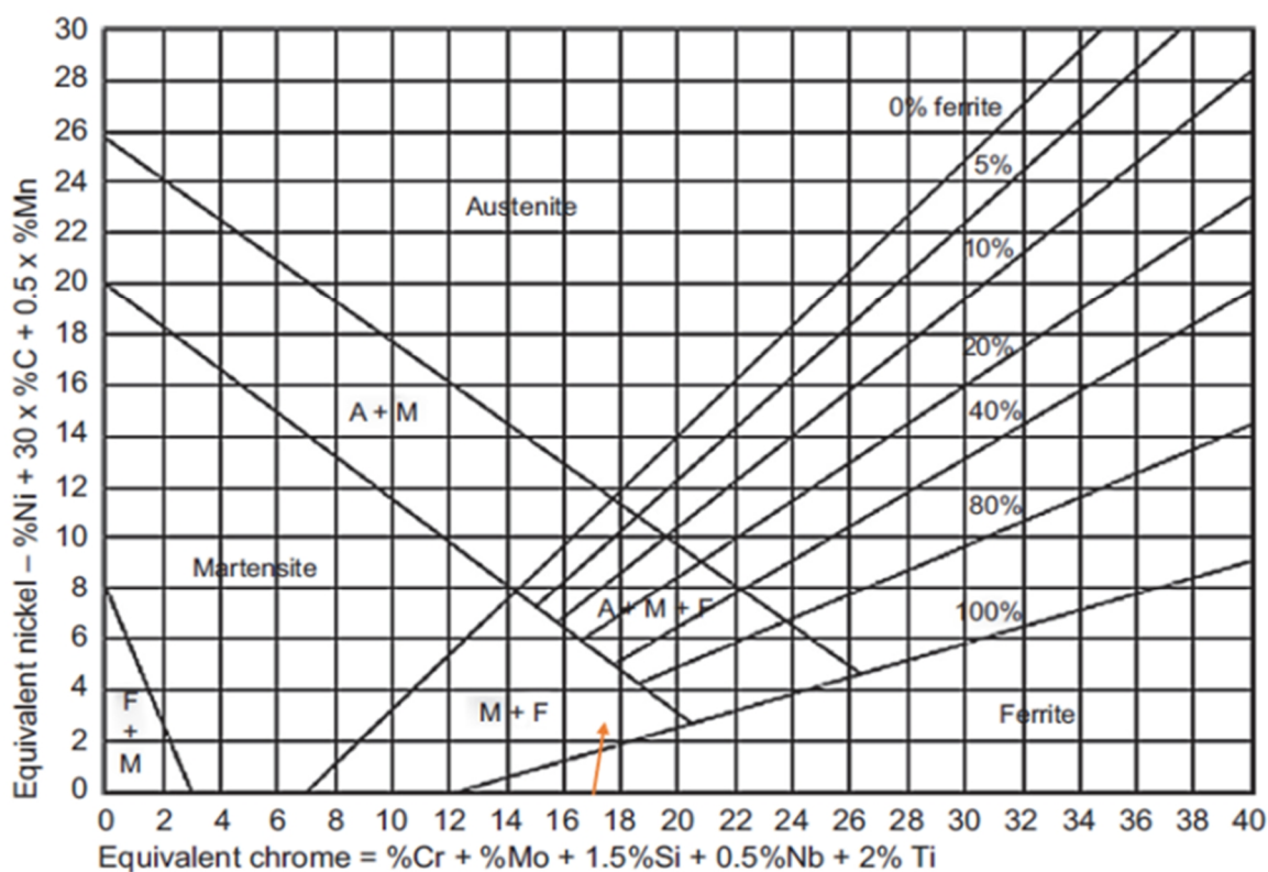
شکل 3- پیش بینی فازهای موجود در فلزجوش براساس مقادیر کروم معادل و نیکل معادل.
