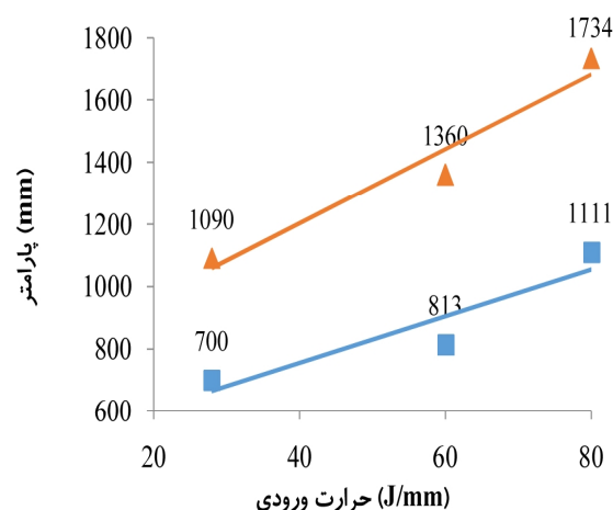
اثر افزایش حرارت ورودی روی عرض و عمق حوضچه مذاب نمودار ۱- عرض جوش عمق جوش
