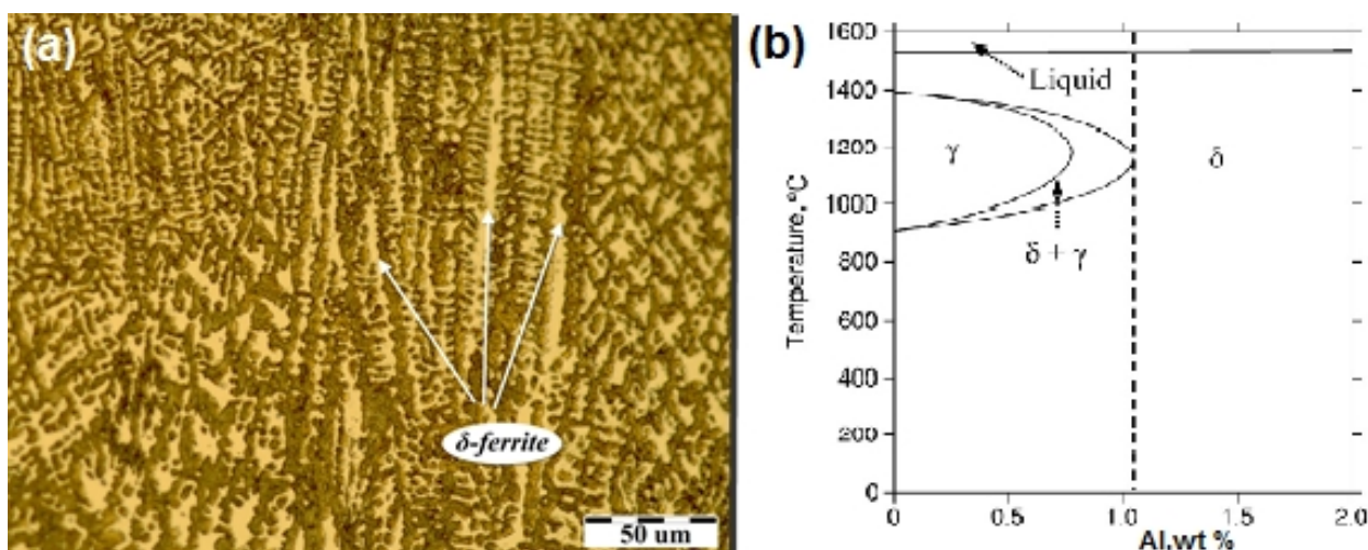
شکل ۴- (a) فاز دندریتی فریت دلتا در منطقه جوش شماره ۳ و (b) دیاگرام تعادلی دوتایی Fe-Al
