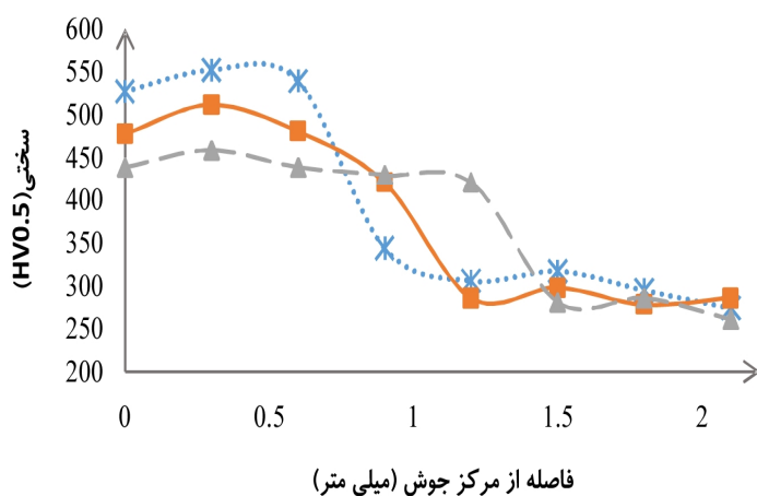
حرارت ورودی 27.9 60 80 نمودار ۲- پروفایل سختی جوش‌ها
