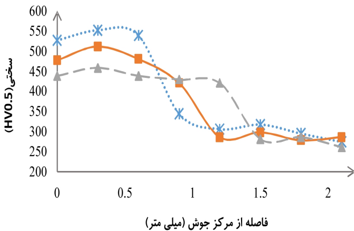
نمودار ۲-پروفایل سختی جوش‌ها حرارت ورودی: 27.9 (نقطه آبی ستاره)، 60 (مربع نارنجی)، 80 (مثلث خاکستری)
