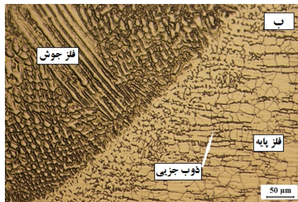
شکل ۱۰- فصل مشترک فلز جوش فولاد 316 L با فلز پایه اینکولوی ۸۲۵ (ا) فصل مشترک فلز جوش فولاد 316 L با فلز پایه فولاد 316 L (ب)
