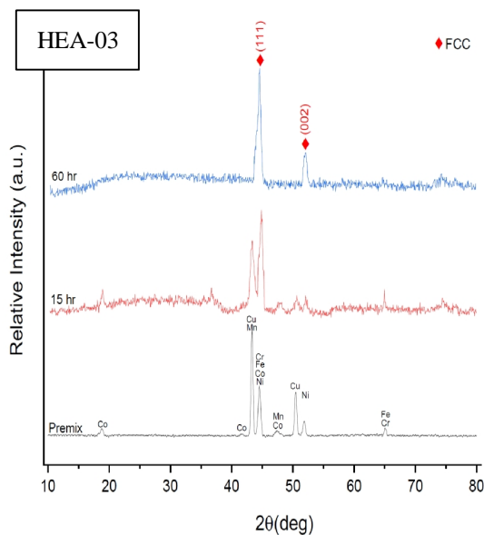
شکل 4- آنالیز XRD سه ترکیب پودر پرکننده.
