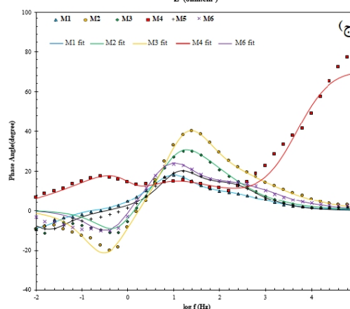
شکل 9-الف - منحنی‌های پلاریزاسیون پتانسیودینامیک، ب - نایکوئیست ( Z' بر حسب Z'' ) حاصل از آزمون EIS، ج - منحنی باد-زاویه فاز نمونه‌های جوشکاری شده نمونه‌های M1 تا M6.
