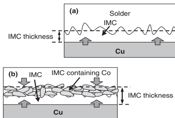
شکل 10- شماتیک رشد ترکیبات بین‌فلزی در فصل مشترک [15].
