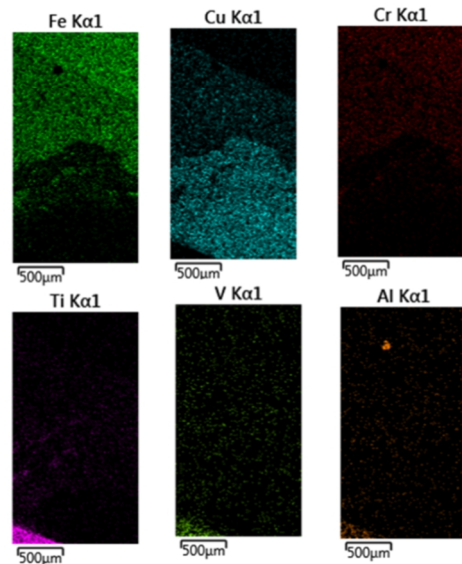
شکل 15- نقشه توزیع عناصر آلیاژی از سطح مقطع اتصال با سرعت 0/9 متر بر دقیقه و انحراف پرتو 0/6 میلی‌متر.
