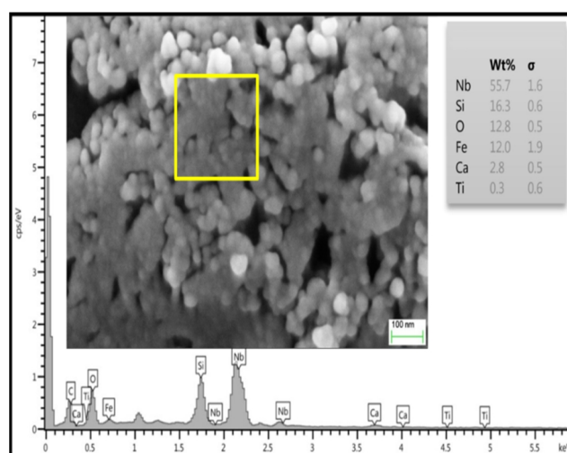
شکل 4- تصویر میکروسکوپ الکترونی روبشی و آنالیز طیف سنگی انرژی اشعه ایکس (EDS) رسوبات حاصل از انحلال فولاد اولیه.
