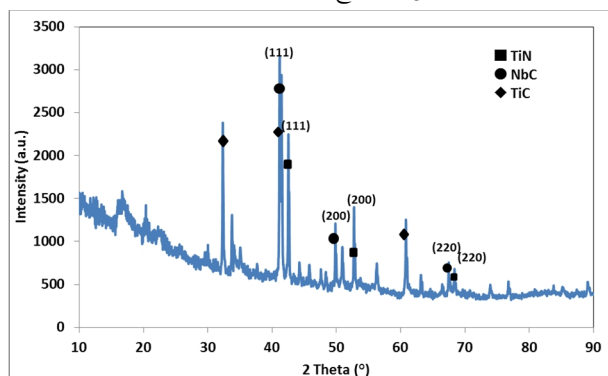
شکل 6- طرح تفرق اشعه X از رسوبات باقی مانده از انحلال شیمیایی فولاد.
