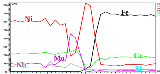
شکل 4- پروفایل توزیع عناصر آلیاژی در امتداد موضع اتصال مجموعه SS-316L/BNi3/IN-625 اتصال داده شده در شرایط: الف - 1150^{\circ}\text{C}/5\text{ min} ، ب - 1150^{\circ}\text{C}/20\text{ min} .
