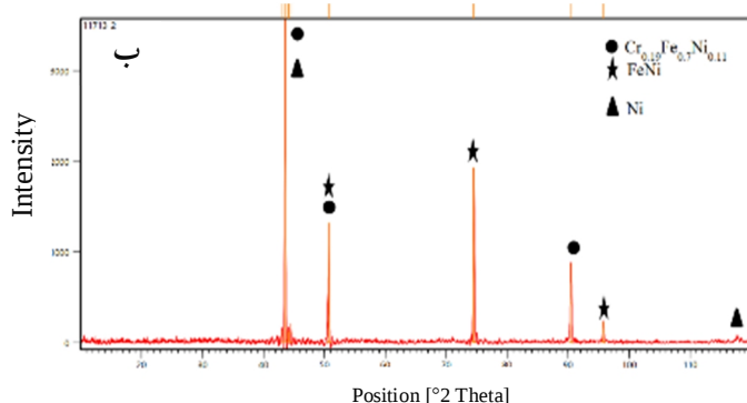
شکل 5- بررسی XRD موضع اتصال. الف - قبل از تکمیل انجماد همدا ( 1050^{\circ}\text{C}/5\text{ min} )، ب - بعد از تکمیل انجماد همدا ( 1050^{\circ}\text{C}/20\text{ min} ).
