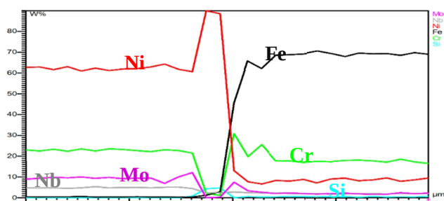
شکل 4- پروفایل توزیع عناصر آلیاژی در امتداد موضع اتصال مجموعه SS-316L/BNi3/IN-625 اتصال داده شده در شرایط: الف - 1150^{\circ}\text{C}/5\text{ min} ، ب - 1150^{\circ}\text{C}/20\text{ min} .
