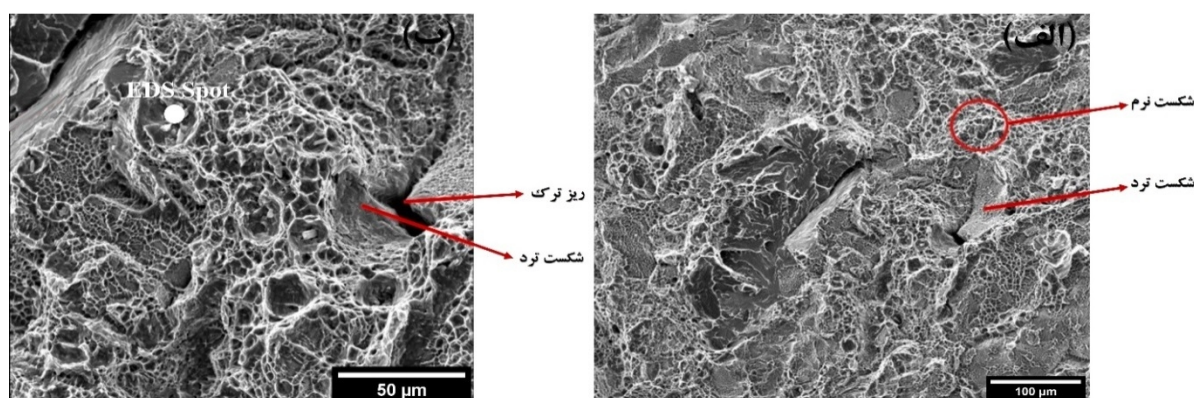
شکل 5- تصویر حاصل از میکروسکوپ الکترونی روبشی (SEM) از مقطع شکست جوش حاصل از فلز پرکننده ER309L بر روی آلیاژ 1/8550 قبل از نیتروژن دهی، الف- بزرگنمایی X 500 و ب- بزرگنمایی X 1500
