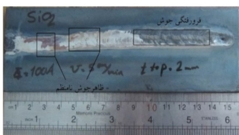
شکل 2- سطح جوش نمونه‌ها الف- تیگ مرسوم ب- نمونه \text{CuO} ج- نمونه \text{MoO}_3 د- نمونه \text{SiO}_2 .
