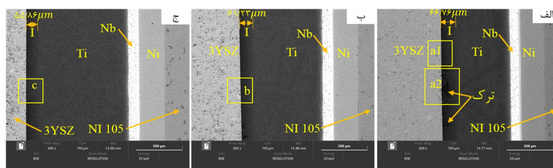
شکل 1- تصاویر FESEM از اتصال 3YSZ/Ti/Nb/Ni/Ni 105 در شرایط مختلف
