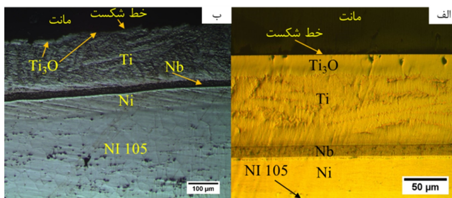
شکل 2- تصاویر میکروسکوپ نوری از اتصالات ناموفق الف- دمای 860°C و زمان 60 دقیقه و ب- دمای 960°C و زمان 30 دقیقه
