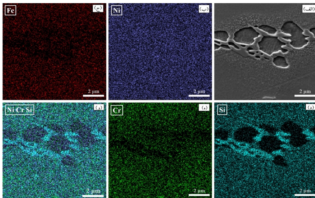
شکل 4- تصاویر الف - SEM و آنالیز نقشه اشعه ایکس (X-ray mapping) عناصر ب - Ni، ج - Fe، د - Si، ه - Cr و و - Ni، Cr، Si از ناحیه اتصال TLP در دمای 1030 °C با زمان نگهداری 30 min
