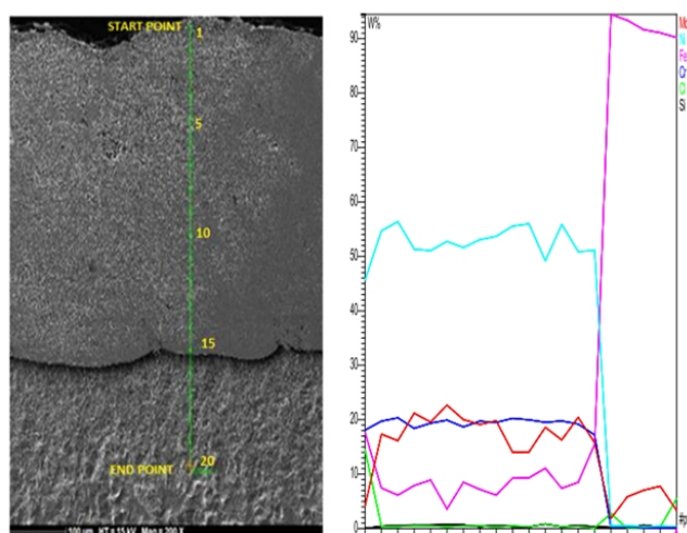
شکل 10- آنالیز عنصری از سطح روکش تا فلزیابه.
