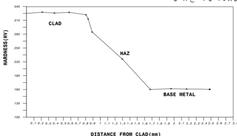
شکل 11- نمودار پروفیل سختی مقطع روکش از سطح آن تا زیرلیه.
