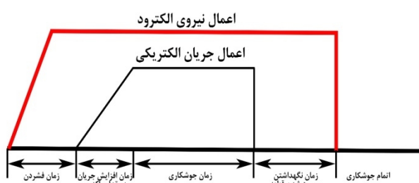
شکل 1- نحوه زمان بندی اعمال نیروی الکتروودها و جریان الکتریکی جهت انجام جوشکاری مقاومتی نقطه‌ای.
