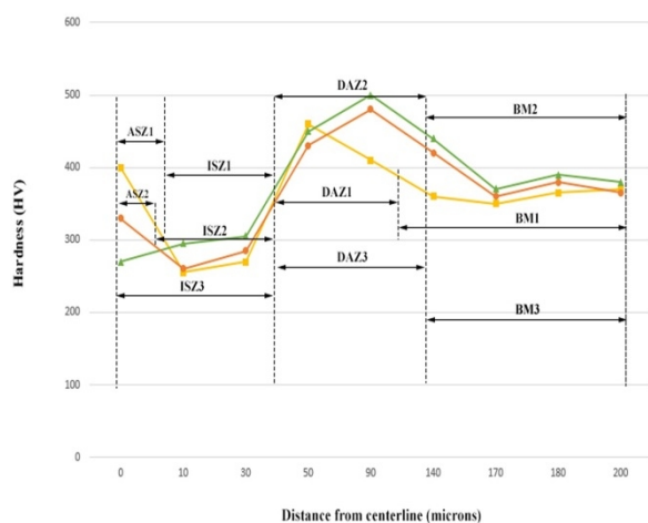
شکل 7- نیمرخ سختی در مناطق مختلف اتصال.
