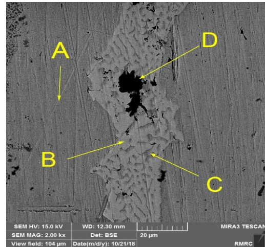
شکل 8 - تصویر میکروسکوپ الکترونی روشنی از محل اتصال نمونه متصل شده در دمای 1120°C و زمان 45 دقیقه. فازهای A, B, C, D در تصویر مشخص هستند که به ترتیب فازهای پرویوتکتیک- \gamma ، بورید غنی از نیکل، یوتکتیک- \gamma و بورید غنی از کروم هستند.
