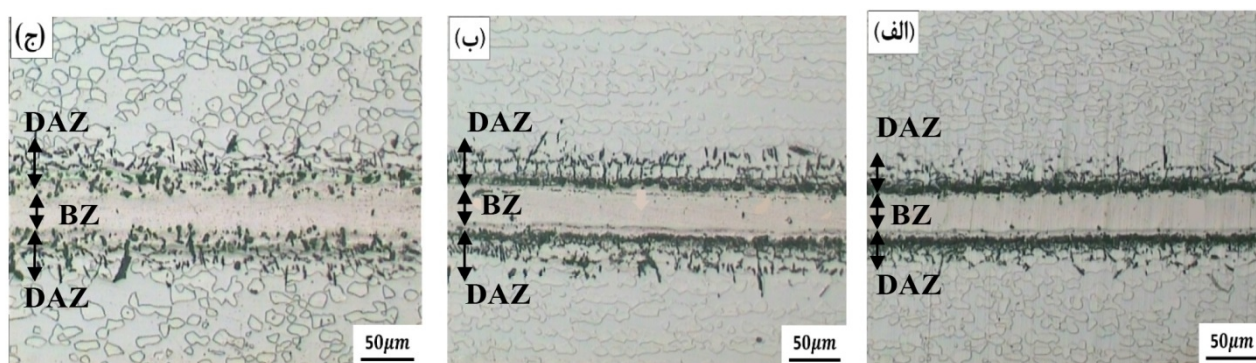
شکل 7- تاثیر دمای اتصال دهی بر ناحیه اتصال TLP ایجاد شده به مدت 20 min در دماهای (الف) 1050 °C، (ب) 1150 °C و (ج) 1200 °C. BZ و DAZ به ترتیب معرف موضع اتصال و موضع متاثر از نفوذ می باشند.
