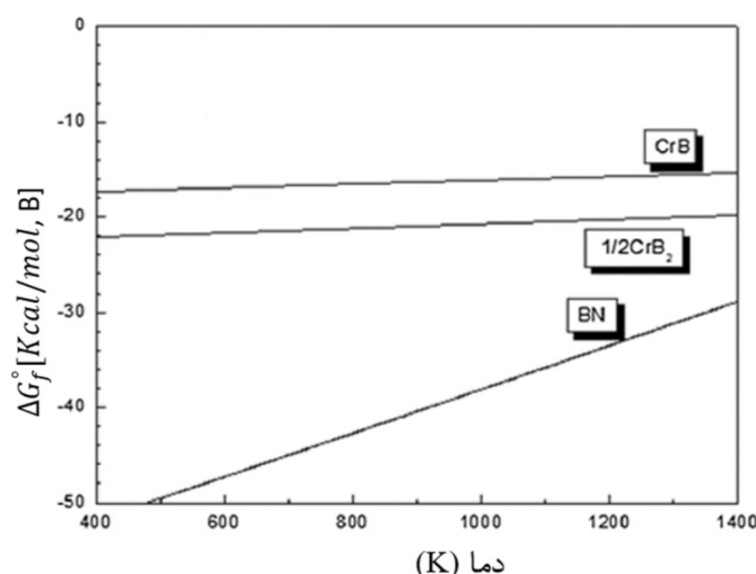
شکل 12- انرژی آزاد استاندارد تشکیل برآیدها و نیتريد ها [28].
